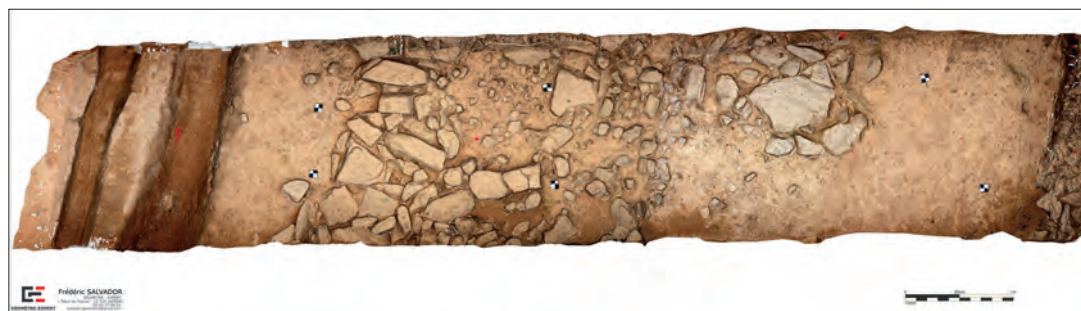
Scan 3D de la voie romaine Tolosa-Segodunum mise au jour près de la route départementale 66 (route de Baraqueville à Luc).
